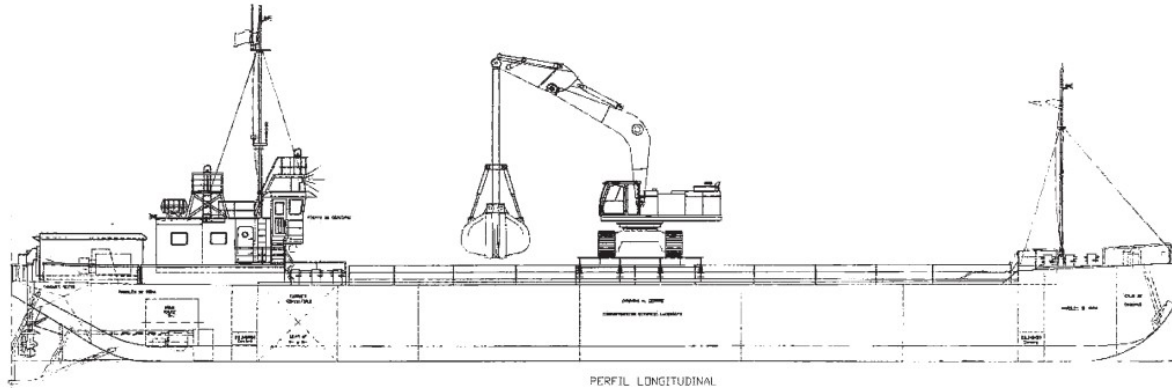
PERFIL LONGITUDINAL
