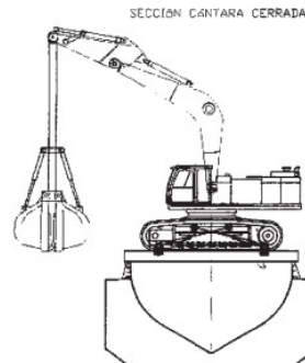
SECCIÓN CÁNTARA CERRADA
