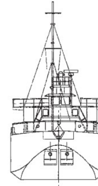
VISTA DE PROA
